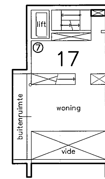
7e verdieping Schaal 1 o 200
